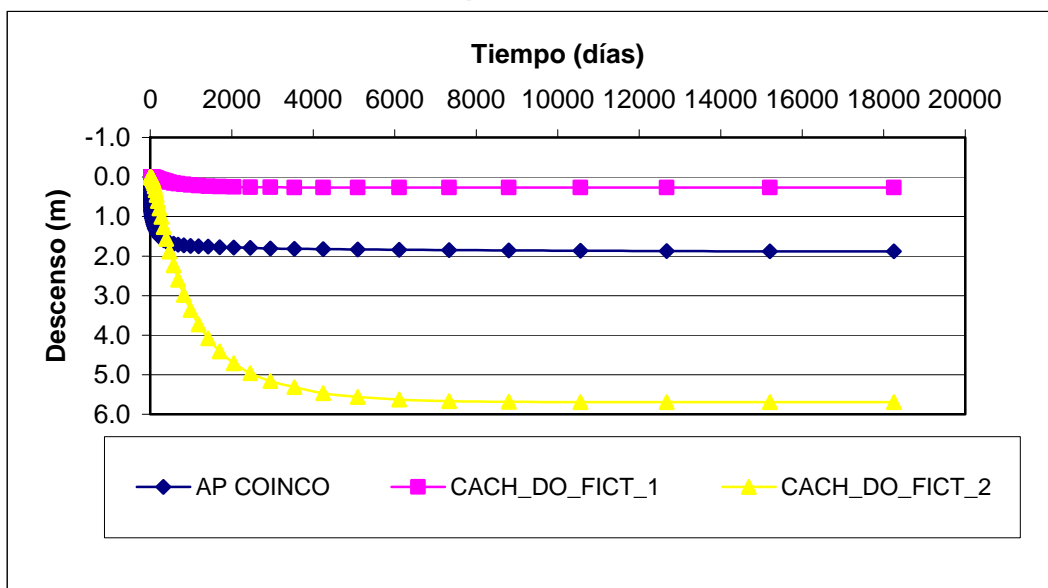
Figura 11 Variación del Nivel de la Napa en Pozos de Observación Sector 4
