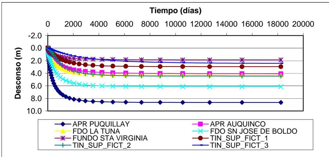
Figura 12 Variación del Nivel de la Napa en Pozos de Observación Sector 2
