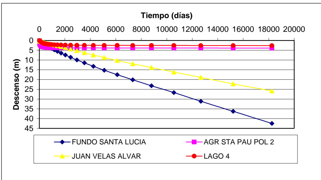
Figura 5 Variación del Nivel de la Napa en Pozos de Observación Sector 3
