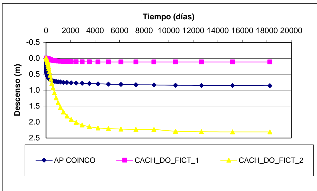
Figura 5 Variación del Nivel de la Napa en Pozos de Observación Sector 4
