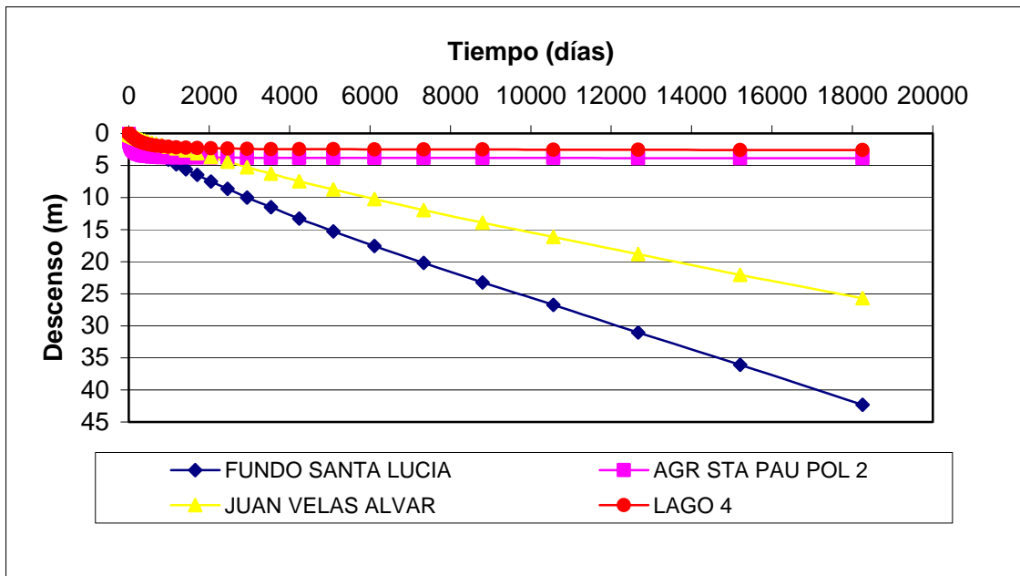
Figura 8 Variación del Nivel de la Napa en Pozos de Observación Sector 3
