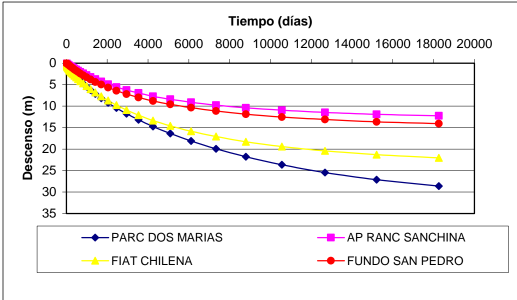
Figura 9 Variación del Nivel de la Napa en Pozos de Observación Sector 2
