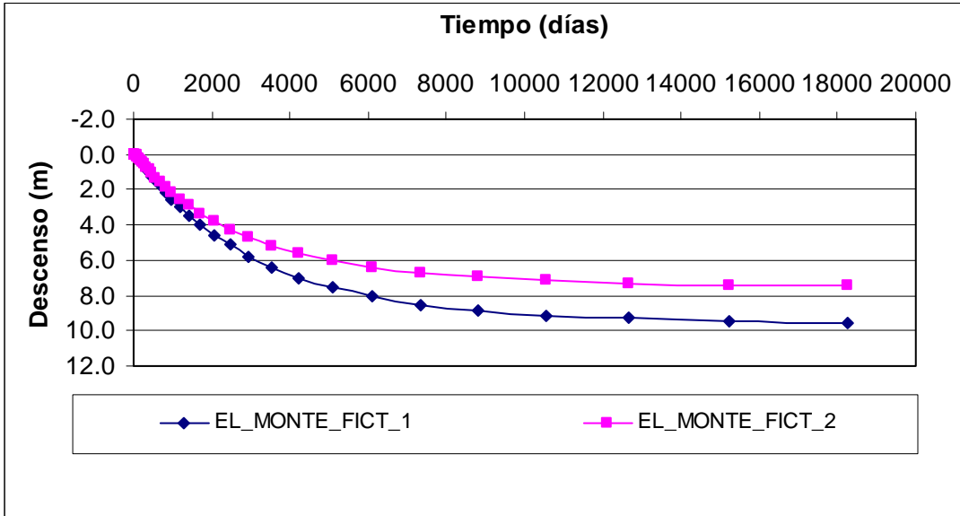
Figura 8 Variación del Nivel de la Napa en Pozos de Observación Sector 6
