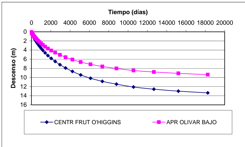
Figura 4 Variación del Nivel de la Napa en Pozos de Observación Sector 3
