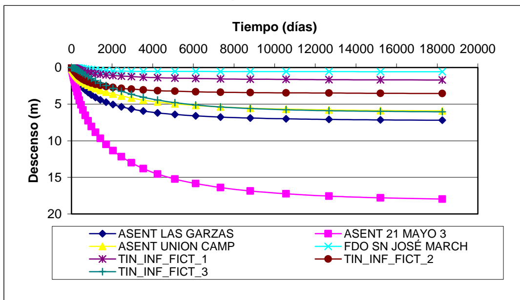
Figura 4 Variación del Nivel de la Napa en Pozos de Observación Sector 1
