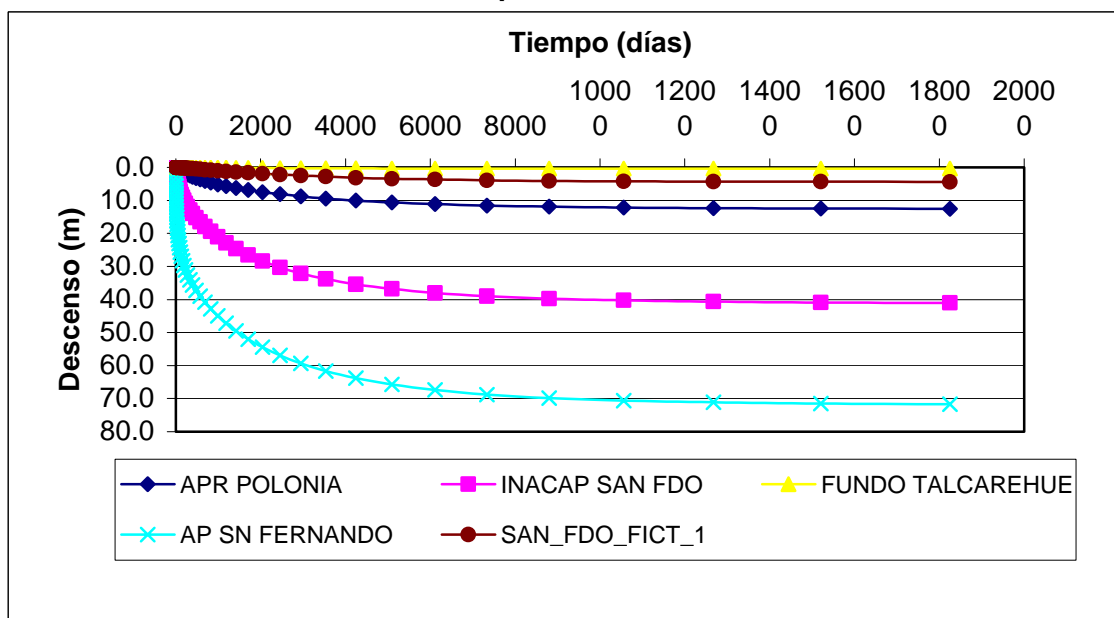
Figura 13 Variación del Nivel de la Napa en Pozos de Observación Sector 3
