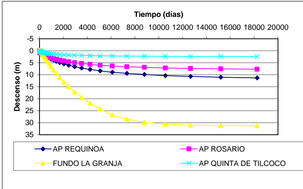
Figura 6 Variación del Nivel de la Napa en Pozos de Observación Sector 5
