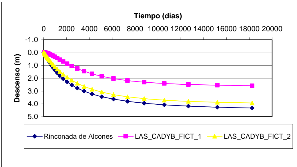
Figura 9 Variación del Nivel de la Napa en Pozos de Observación Sector 7
