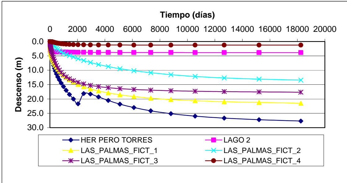
Figura 7 Variación del Nivel de la Napa en Pozos de Observación Sector 2
