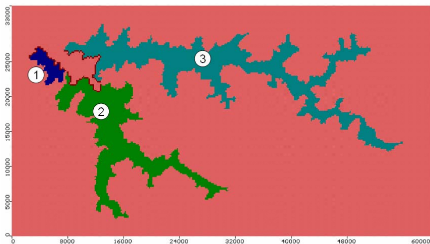
Figura 1 Sectores de Balance Modelados en la Cuenca del Río Alhué
