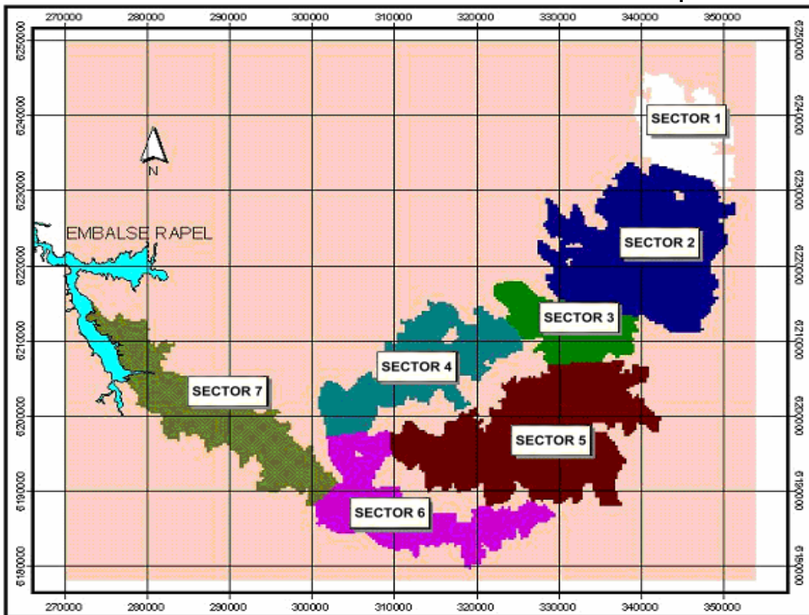
Figura 1 Sectores de Balance Modelados en la Cuenca del Río Cachapoal
