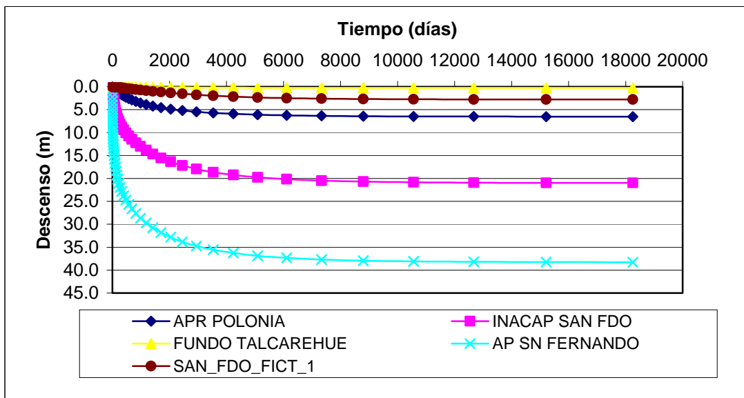
Figura 6 Variación del Nivel de la Napa en Pozos de Observación Sector 3
