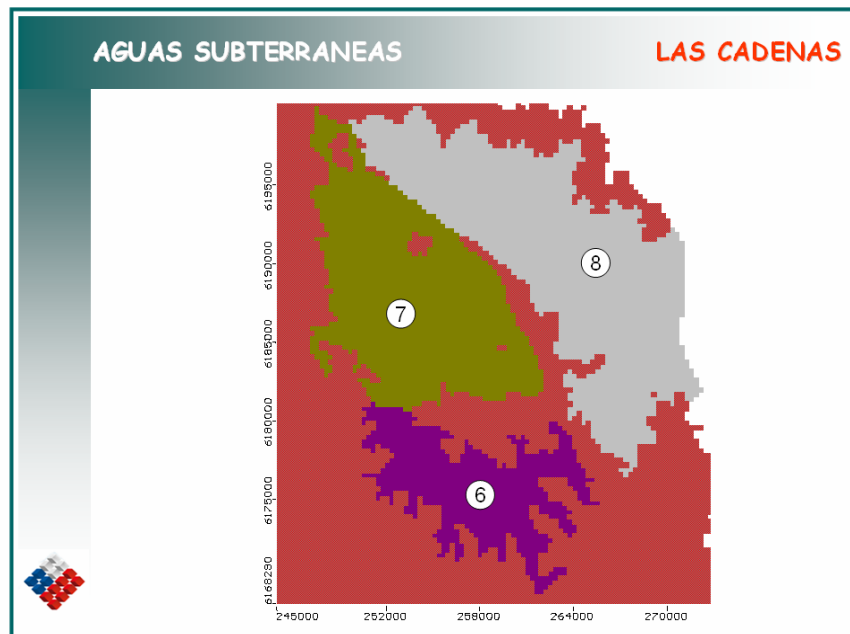
Figura 2 Sectores de Balance Disgregación Sector 5
