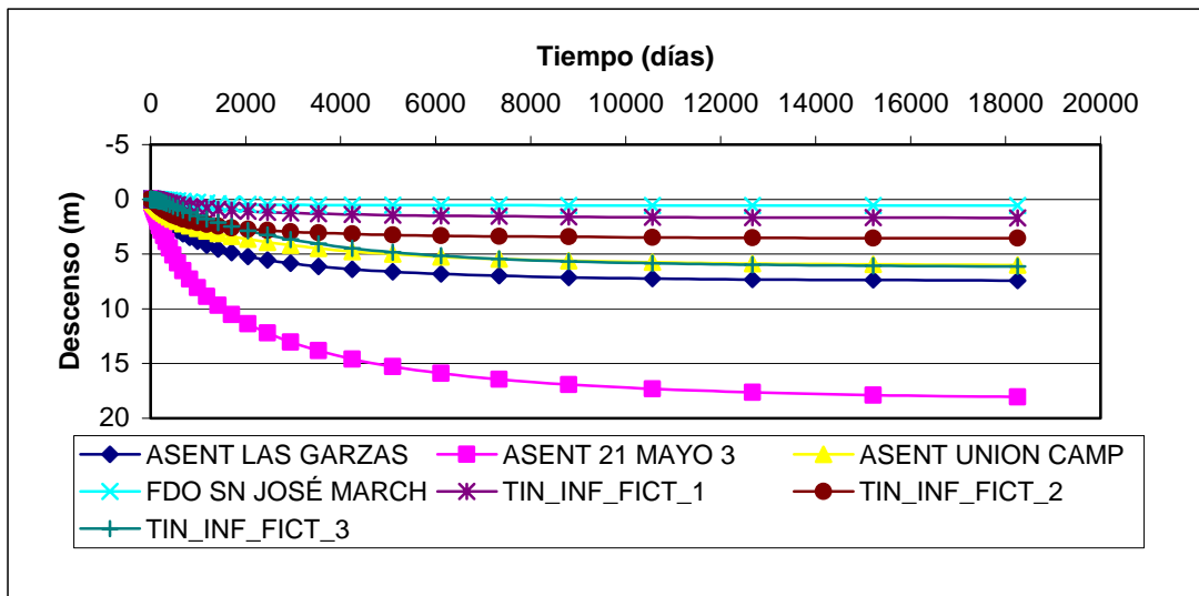
Figura 11 Variación del Nivel de la Napa en Pozos de Observación Sector 1
