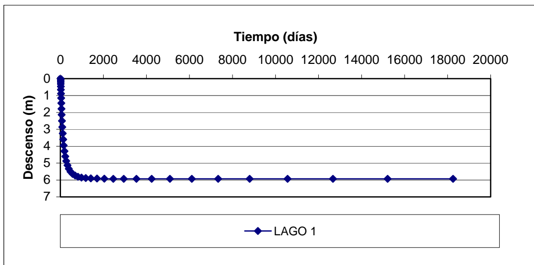
Figura 6 Variación del Nivel de la Napa en Pozos de Observación Sector 1
