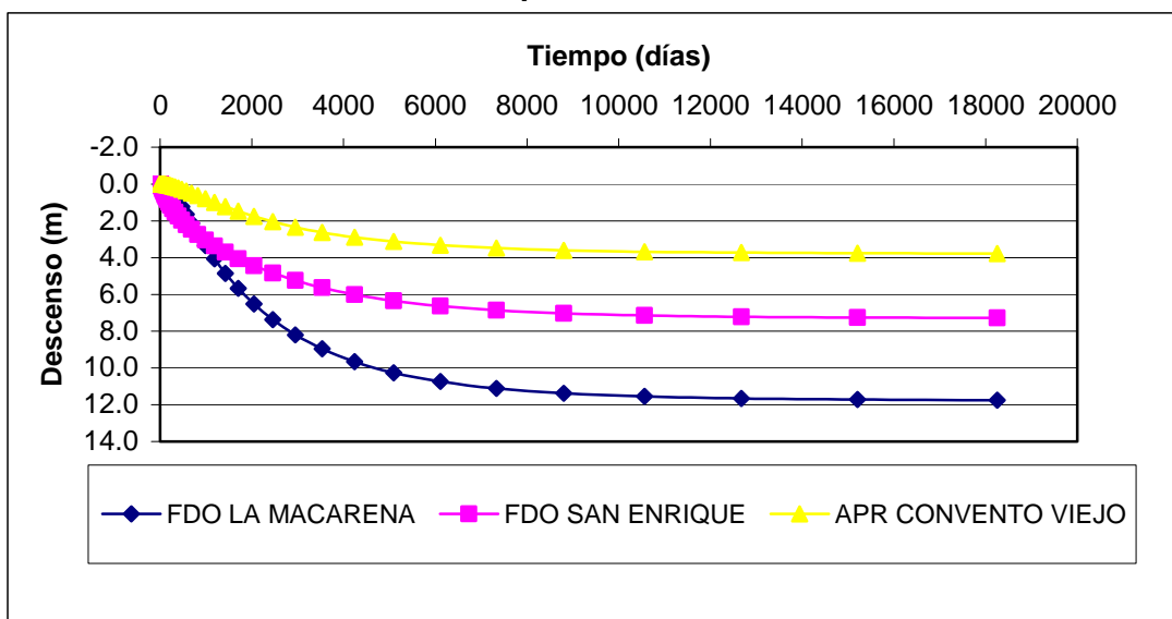
Figura 7 Variación del Nivel de la Napa en Pozos de Observación Sector 4
