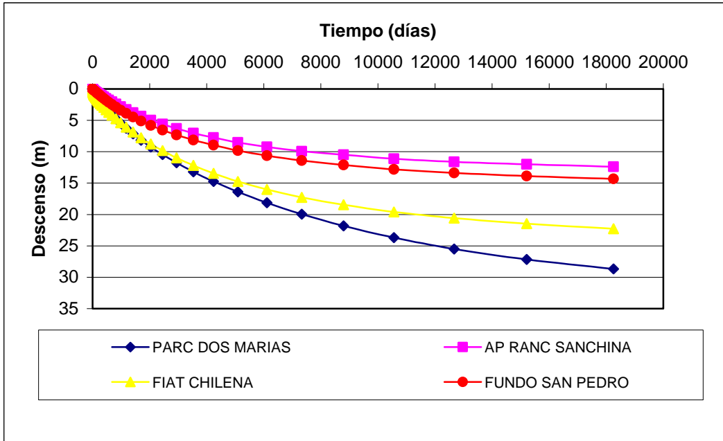
Figura 3 Variación del Nivel de la Napa en Pozos de Observación Sector 2
