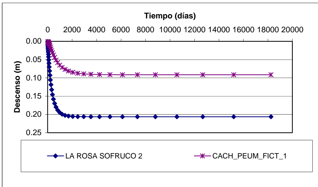
Figura 8 Variación del Nivel de la Napa en Pozos de Observación Sector 7
