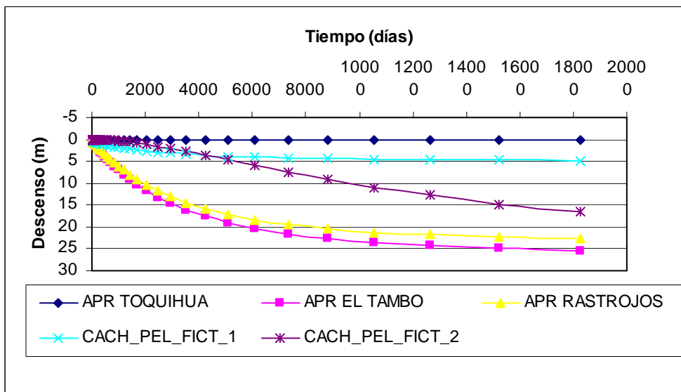
Figura 7 Variación del Nivel de la Napa en Pozos de Observación Sector 6
