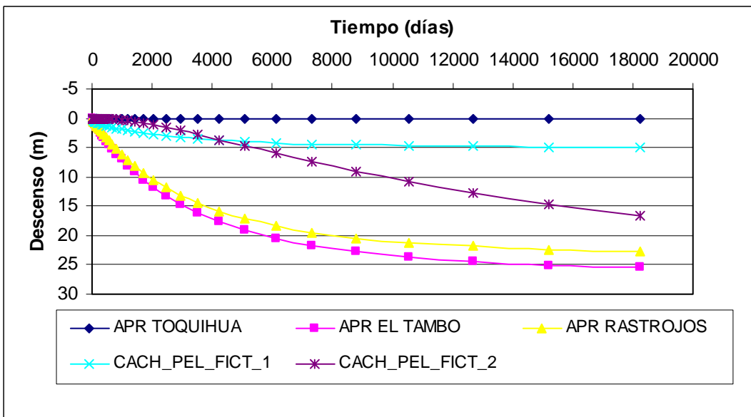
Figura 13 Variación del Nivel de la Napa en Pozos de Observación Sector 6
