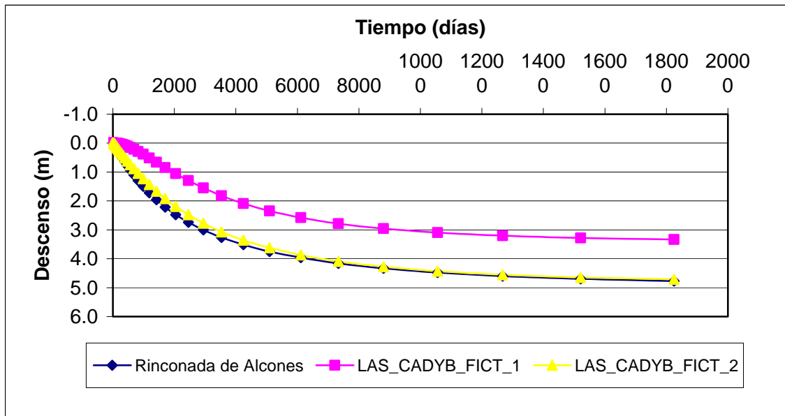
Figura 16 Variación del Nivel de la Napa en Pozos de Observación Sector 7
