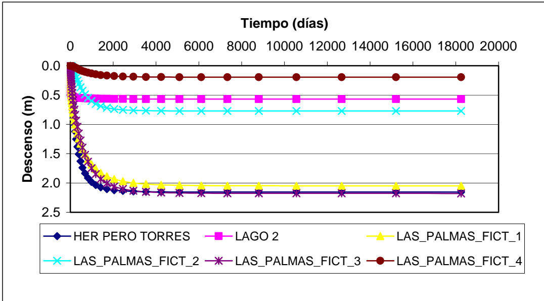
Figura 4 Variación del Nivel de la Napa en Pozos de Observación Sector 2
