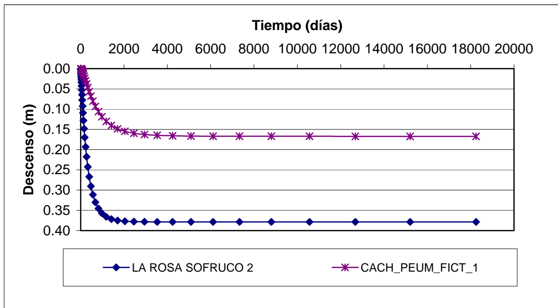
Figura 14 Variación del Nivel de la Napa en Pozos de Observación Sector 7
