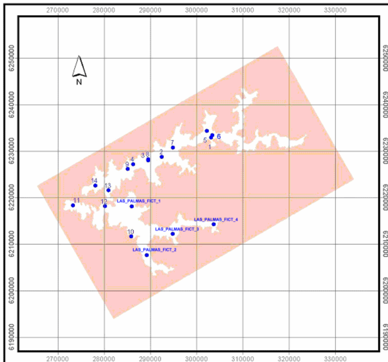
Figura 2 Ubicación de Pozos de Observación Analizados
