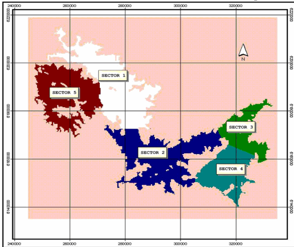
Figura 1 Sectores de Balance Modelados en la Cuenca del Río Tinguiririca
