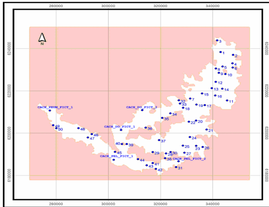
Figura 2 Ubicación de Pozos de Observación Analizados
