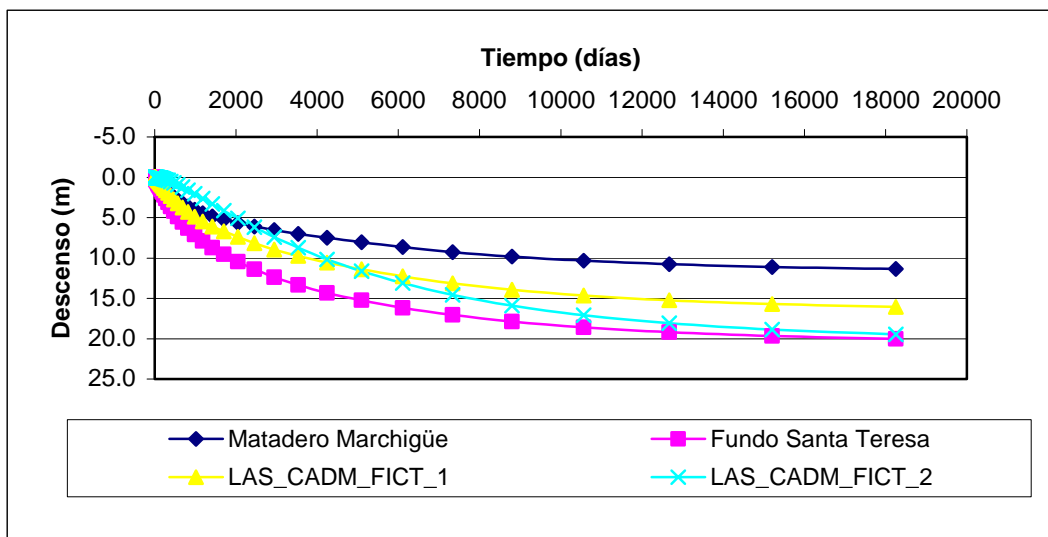
Figura 17 Variación del Nivel de la Napa en Pozos de Observación Sector 8
