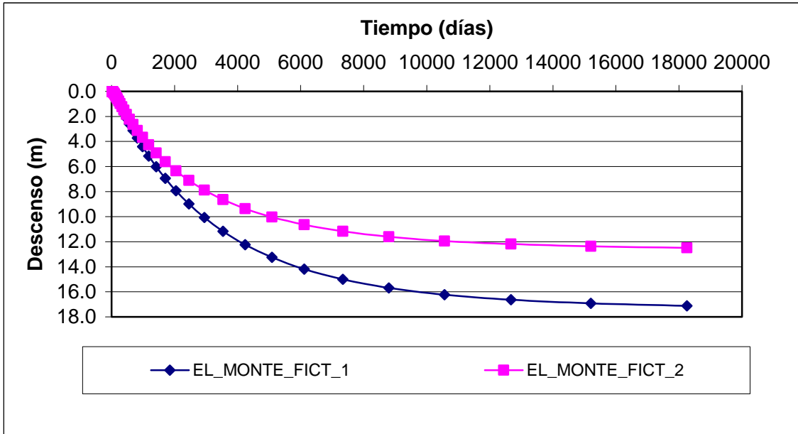
Figura 15 Variación del Nivel de la Napa en Pozos de Observación Sector 6
