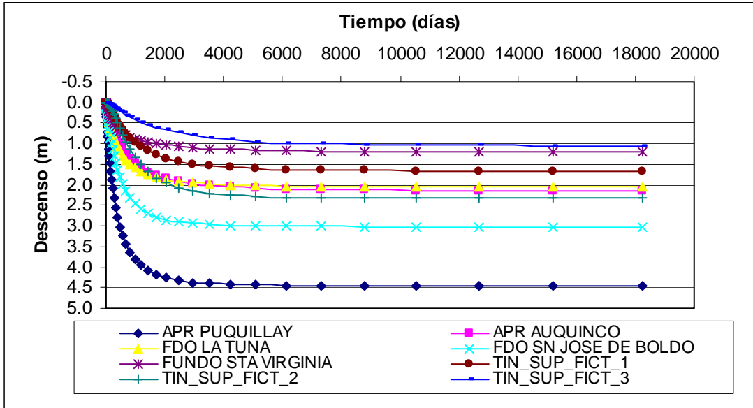
Figura 5 Variación del Nivel de la Napa en Pozos de Observación Sector 2
