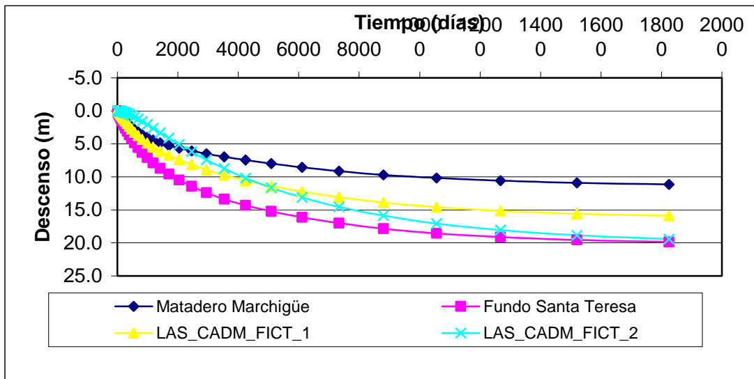
Figura 10 Variación del Nivel de la Napa en Pozos de Observación Sector 8
