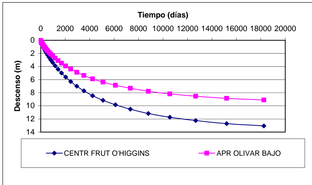
Figura 10 Variación del Nivel de la Napa en Pozos de Observación Sector 3
