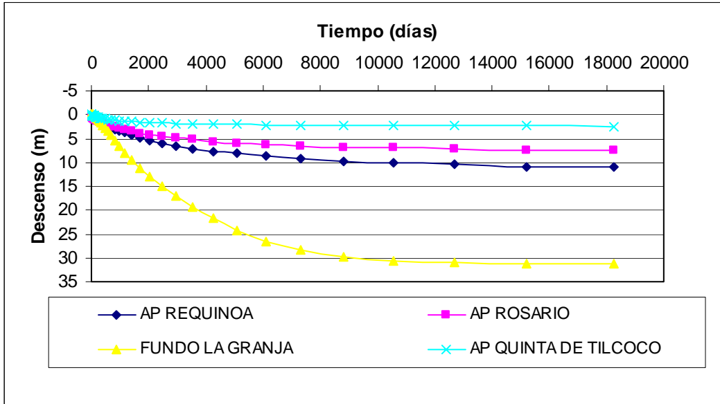
Figura 12 Variación del Nivel de la Napa en Pozos de Observación Sector 5
