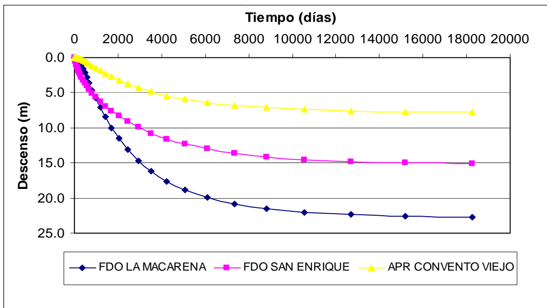
Figura 14 Variación del Nivel de la Napa en Pozos de Observación Sector 4
